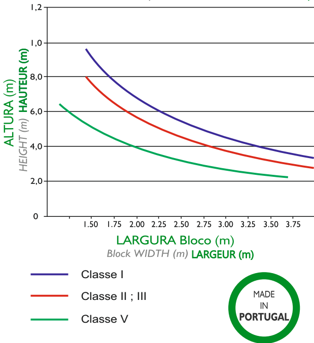
Parâmetros de corte Cut parameters Paramètres de coupe
